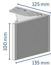
Profilé d'angle 100 mm
